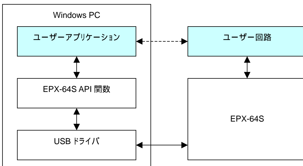
図 1 構成
