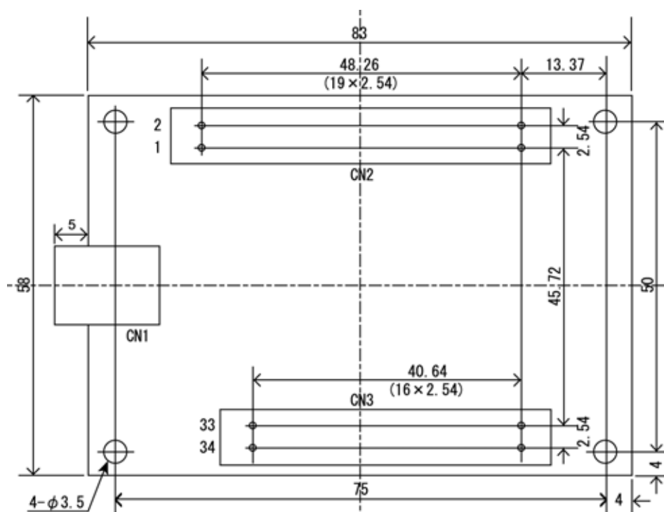
図 2.3 外形寸法
